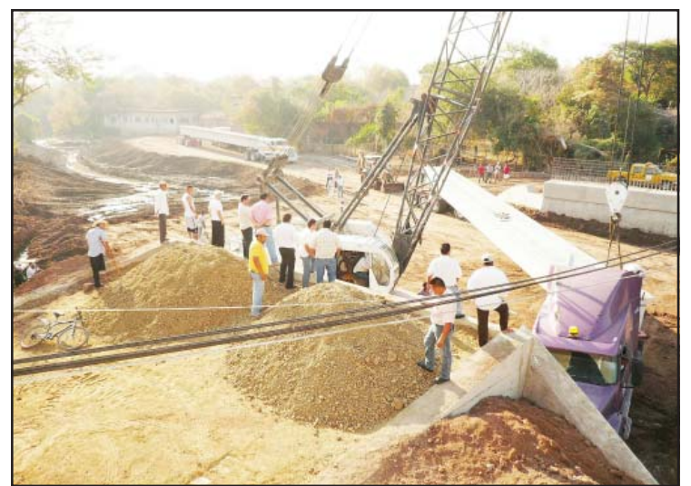
El presidente municipal de Huetamo, Roberto García Sierra, acompañado por funcionarios municipales y trabajadores de la obra, presenciaron las maniobras de la "pluma" para colocar la primera trabe de lo que será el puente.
